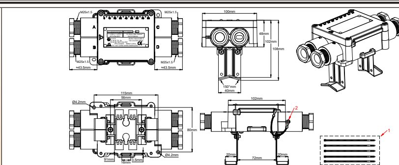
Ejemplo de montaje a distancia de la tubería con soporte de patas largas de acero inoxidable (opción de montaje 5)
