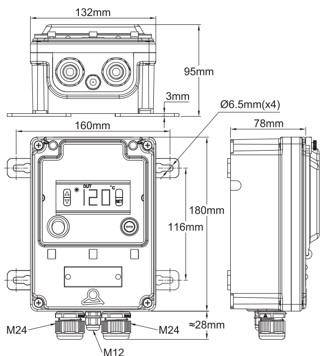
Modelo con 3 glándulas de cable (2 x M24 + 1 x M12): Y8WH-X
