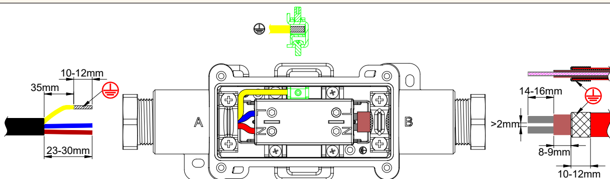
Modelo con un cable de alimentación y un cable calefactor
